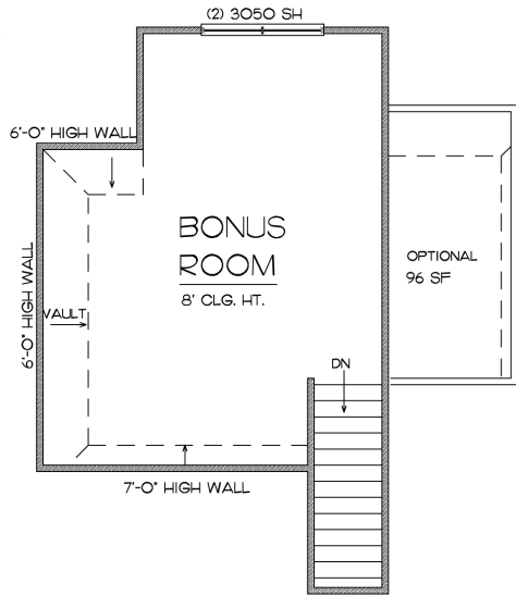
PLAN 2170
